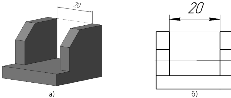
Рис. 52.1. Линейный размер в модели (а) и соответствующий ему проекционный размер в ассоциативном виде (б)
